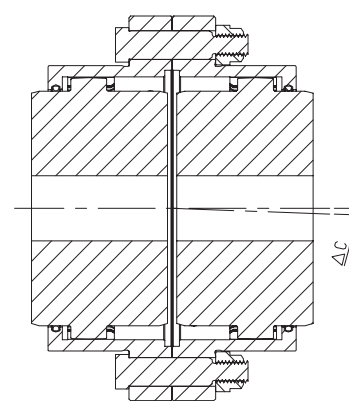
Desalineamiento Angular
