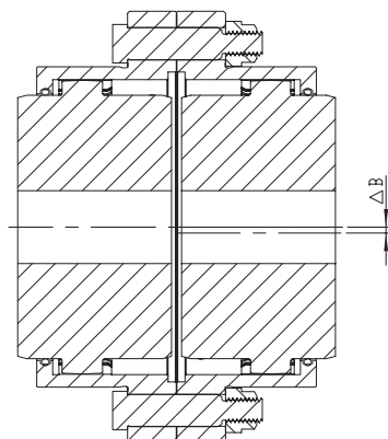
Desalineamiento Paralelo
